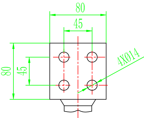
低压接线端子
