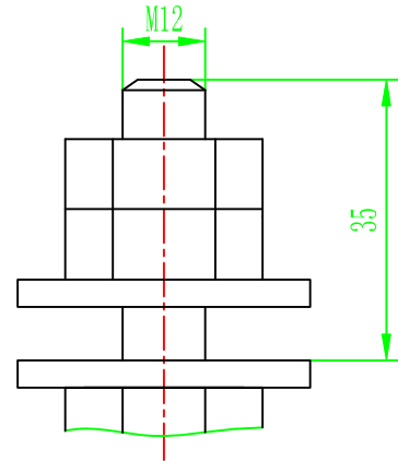
高压套管接线端子
